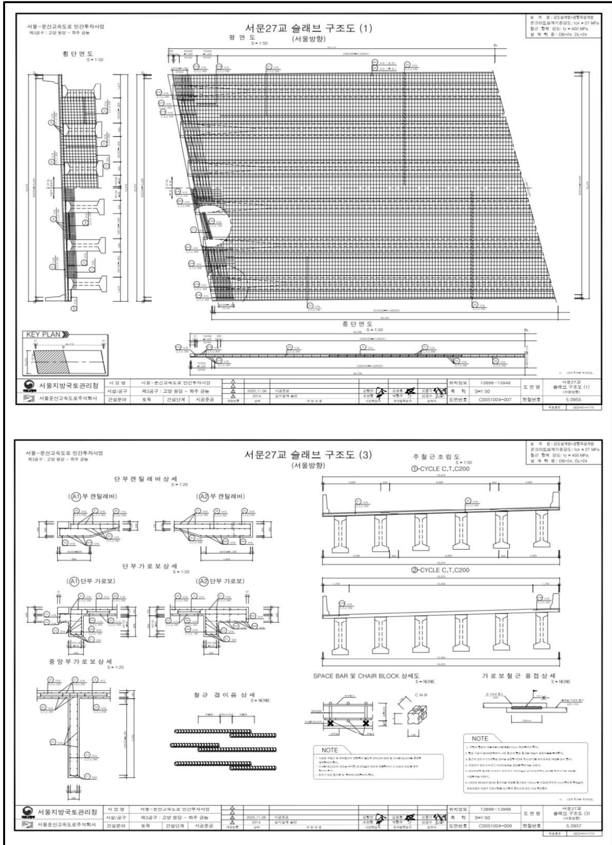
【그림 29.1.6】 바닥판하면 배근도
